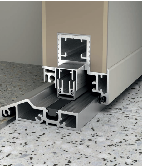
Seuil aluminium avec joint escamotable automatique standard (sans plus value)
